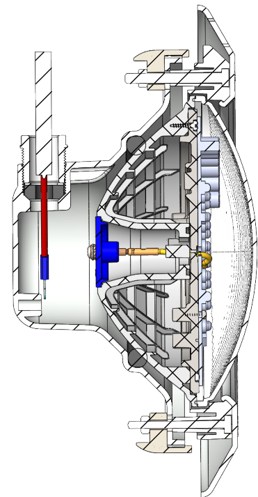
SECCIÓN A-A
